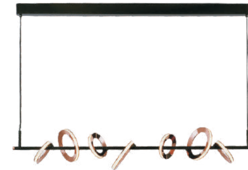
# 6379S-L7-LED 吊钩 pendant lamp ⌀122*17*150cm 灯 - 材料 Aluminum alloy / carbon steel 颜色 Black+rose gold
